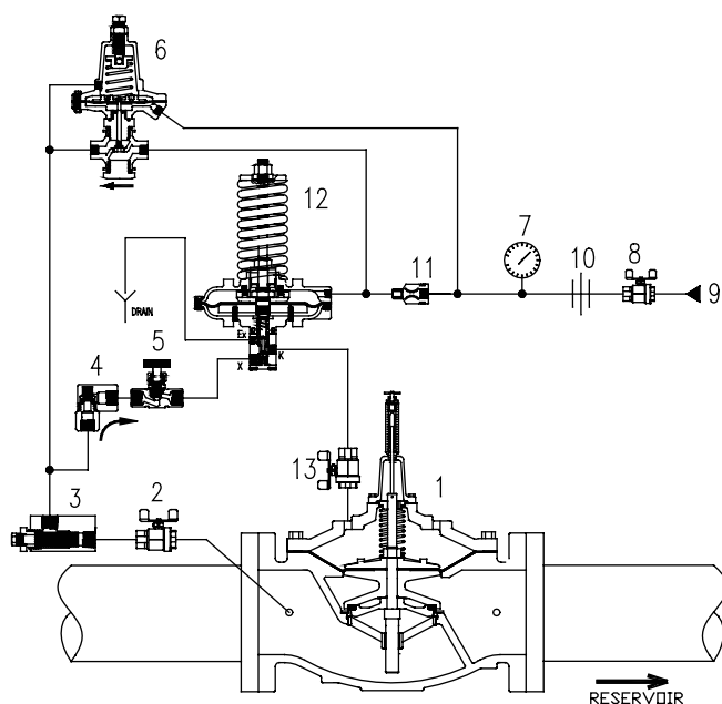
Schematic A-0414D
